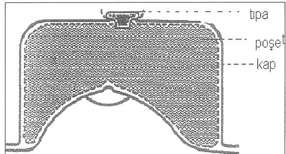
Şekil 4. E. Tezel ve arkadaşlarının hacim ölçme düzeneği.
